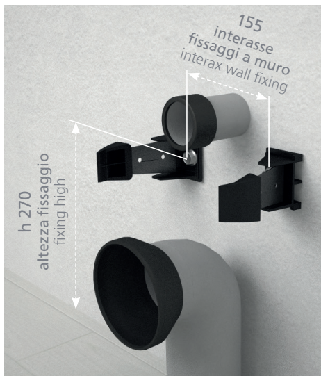
Y1DR fissaggio nascosto per vasi e bidet filo muro senza fori laterali blind fixing for back to wall wc and bidet without side holes
